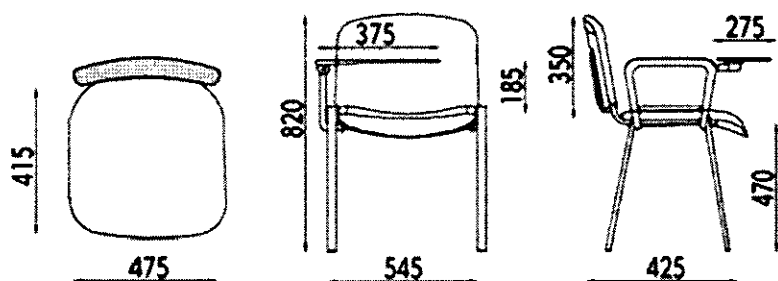
Rys. 3. Wymiary krzesła w ujęciu graficznym. (Poz. 4 specyfikacji przetargowej)
