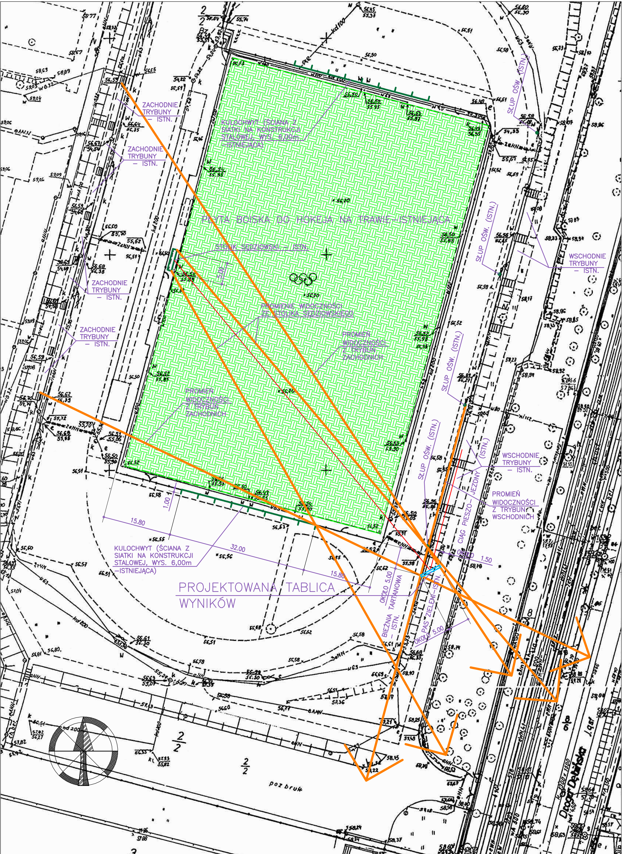
TABLICA WYNIKÓW DO HOKEJA NA TRAWIE - AWF POZNAŃ PLAN SYTUACYJNY, SKALA 1:500 PRACE PRZEDPROJEKTOWE
